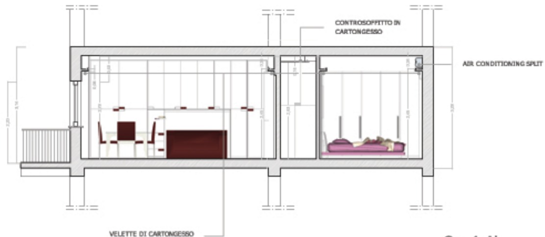
Sez A-A' scala 1:100
